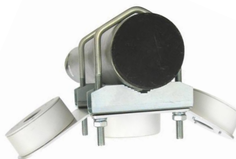
HIK100E TRIO + 2x Z5V105 montáž na trubku (Ø 90mm)
