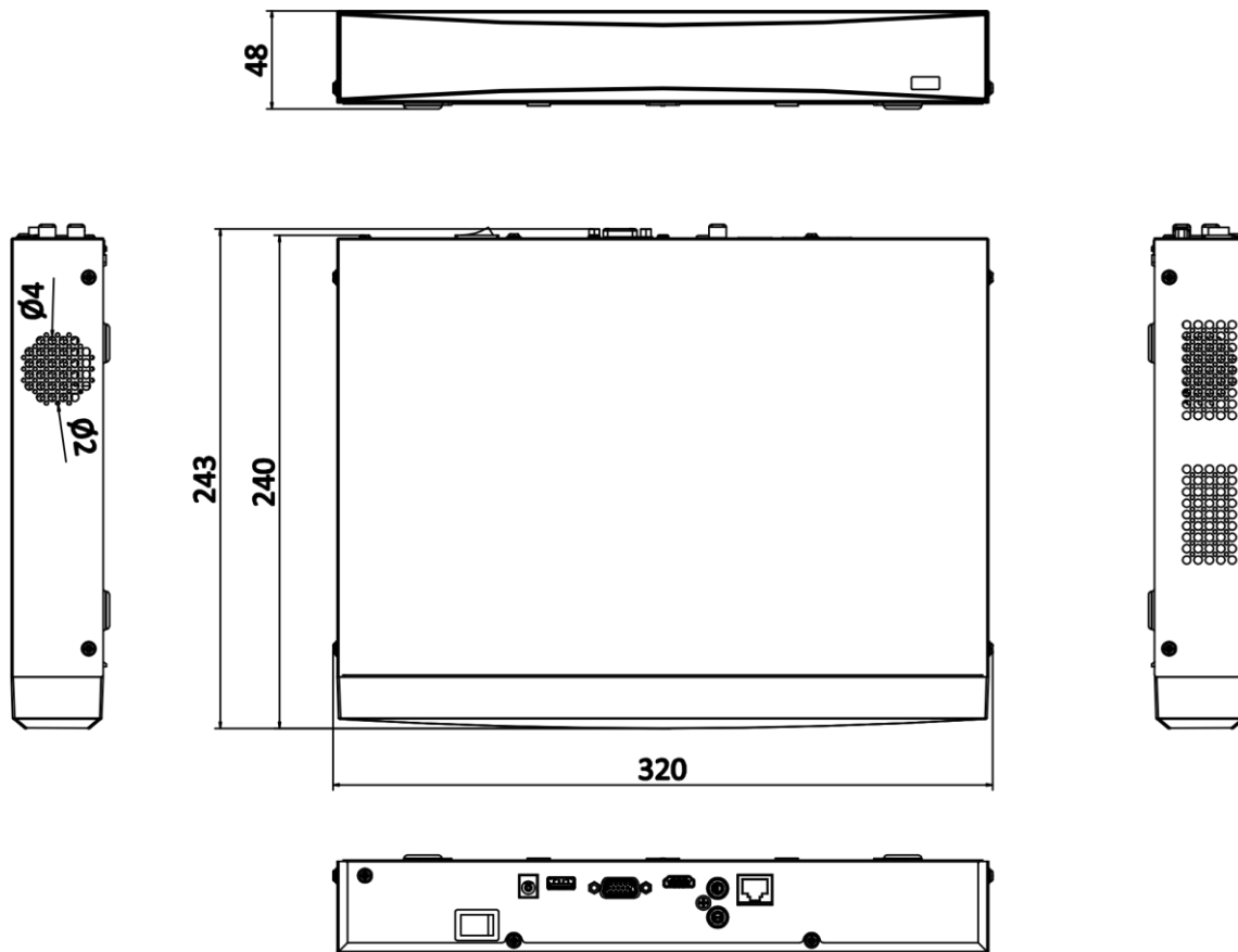
scale/1:1;Unit/mm
